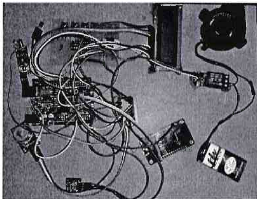
Fig(a):Helmet Module
